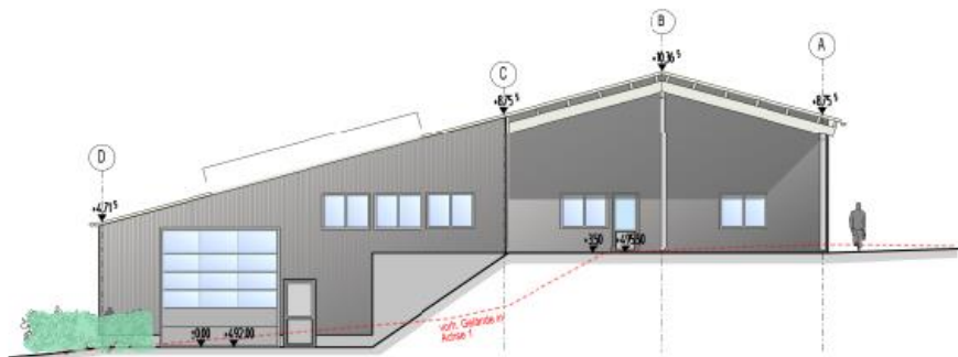
Ansicht Westen
