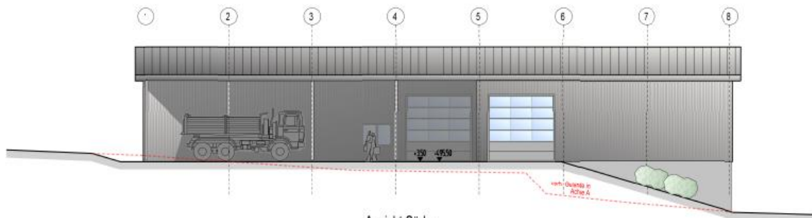
Ansicht Süden
